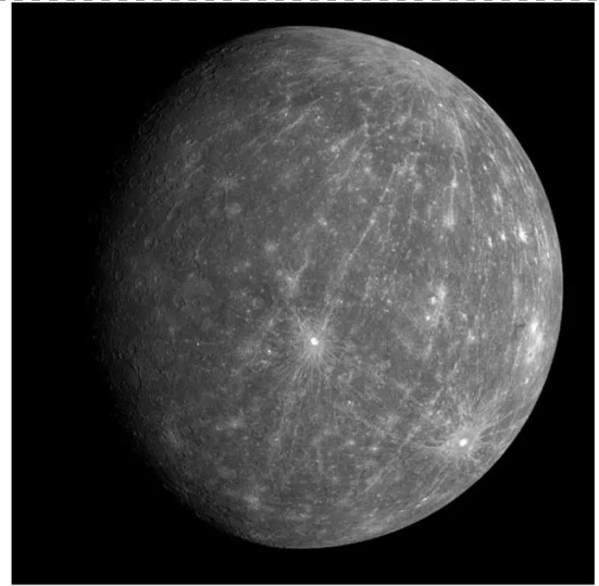
mercurius
