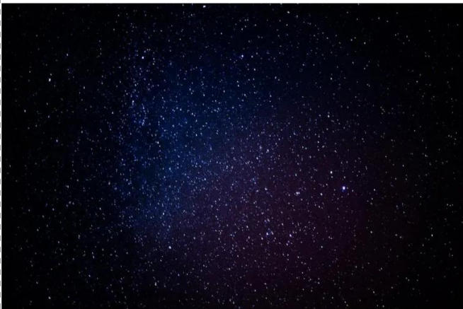
sterrehemel
