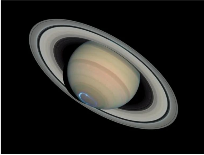
saturnus
