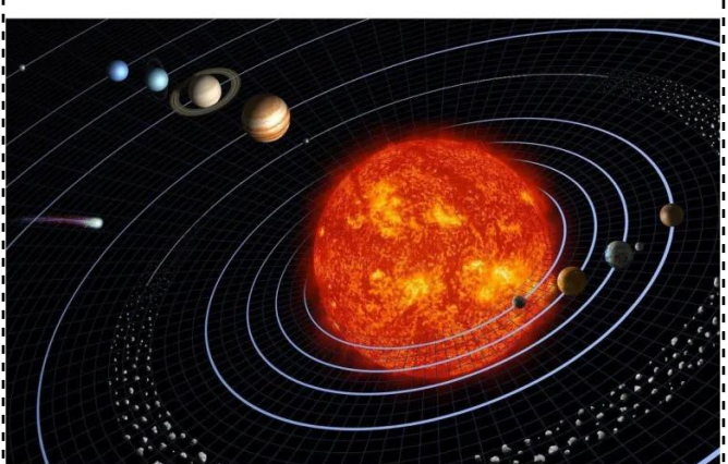
sonnestelsel
