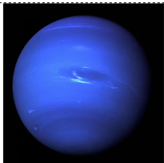
neptunus
