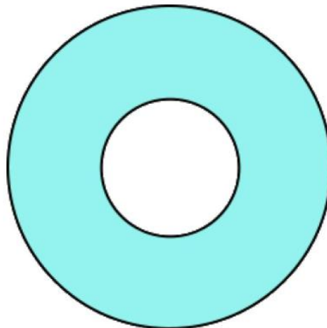
annulus
