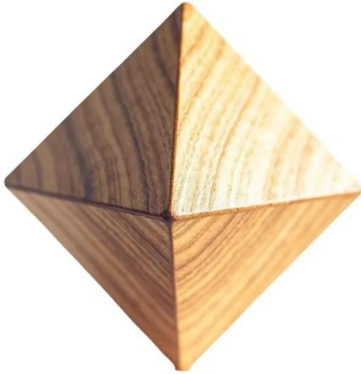
octaedru
